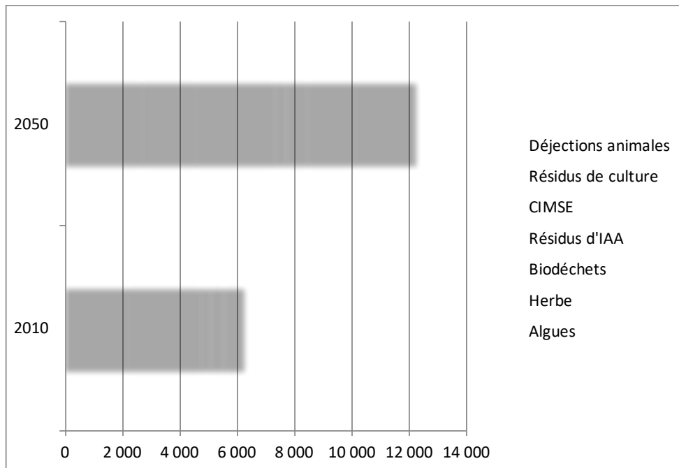
Figure 23 : Potentiel de production de la méthanisation comparé : 2010 et 2050 (GWh PCs)
