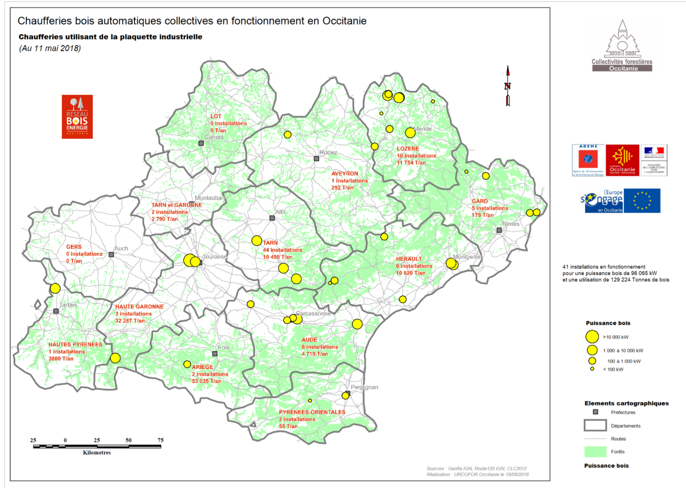
Figure 8 : Chaufferies bois utilisant de la plaquette industrielle en fonctionnement en Occitanie (Source UR COFOR Occitanie)
